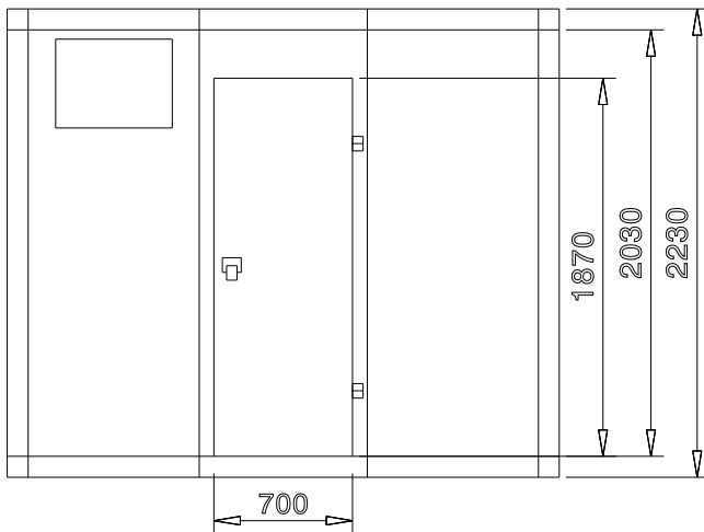
Zij aanzicht
