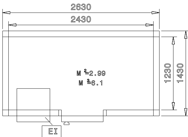
Zij aanzicht
